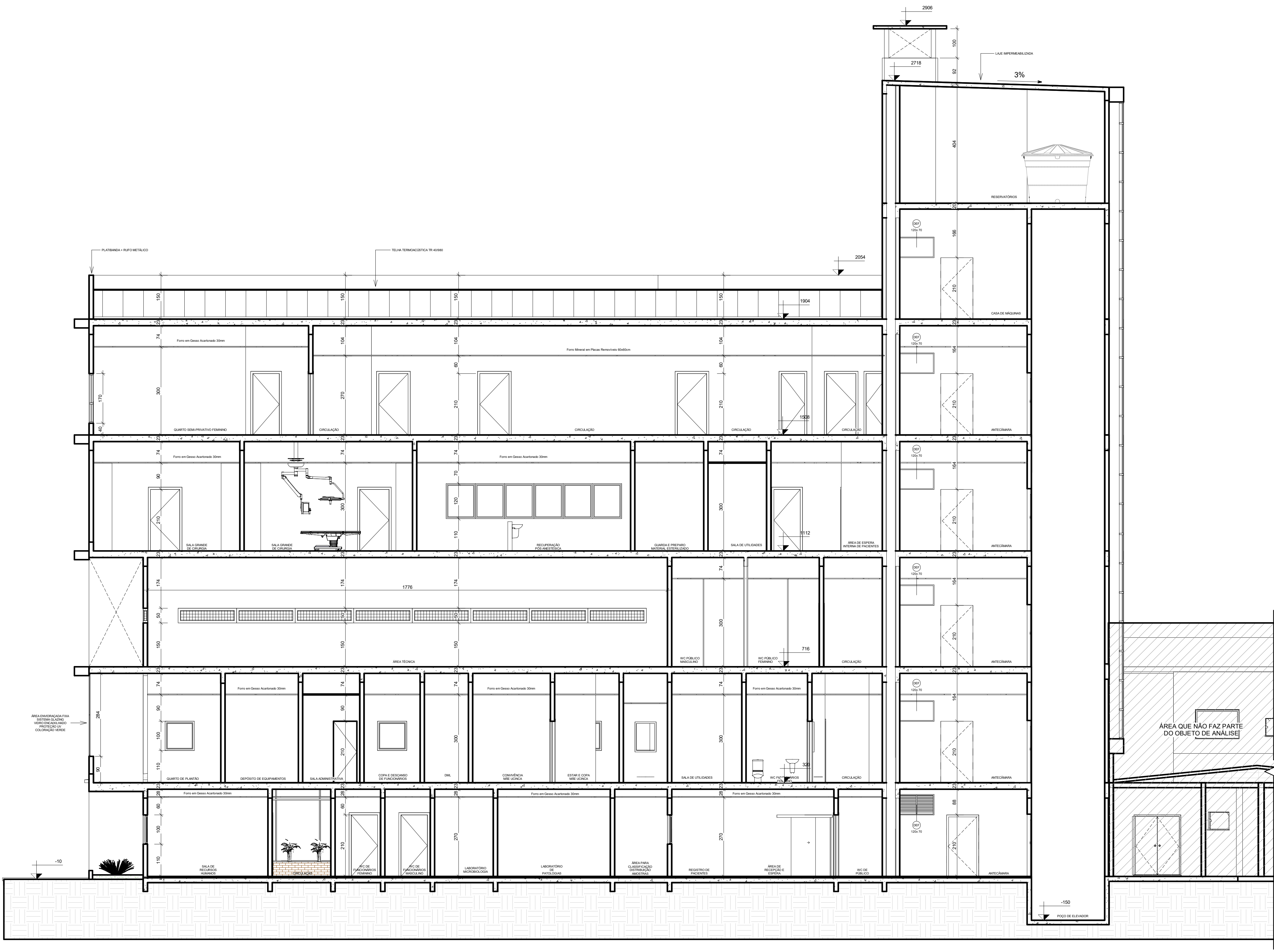
25 CORTE A 1:75
